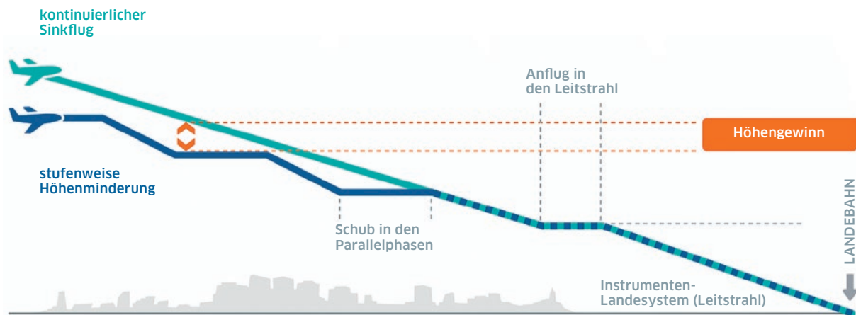
Abb. 6: Sinkflug-Darstellung | © Flughafenverband ADV (Quelle: www.fluglärm-portal | Deutsche Flugsicherung)
