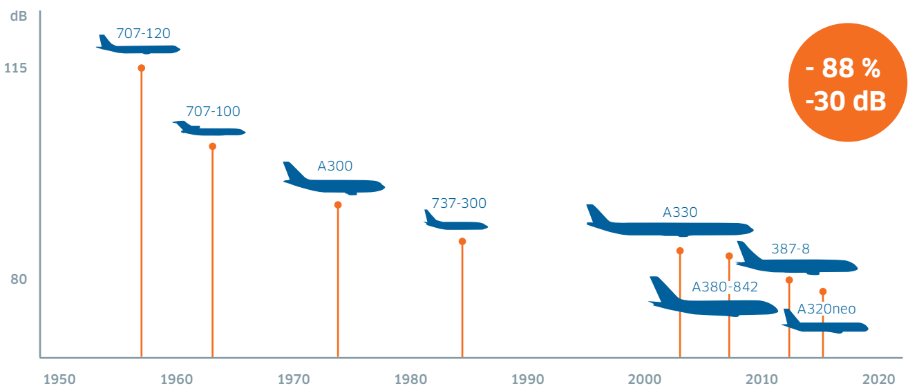
Abb. 2: Seitenlinienpegel normiert auf 500 kN (EPNdB) | © Flughafenverband ADV
